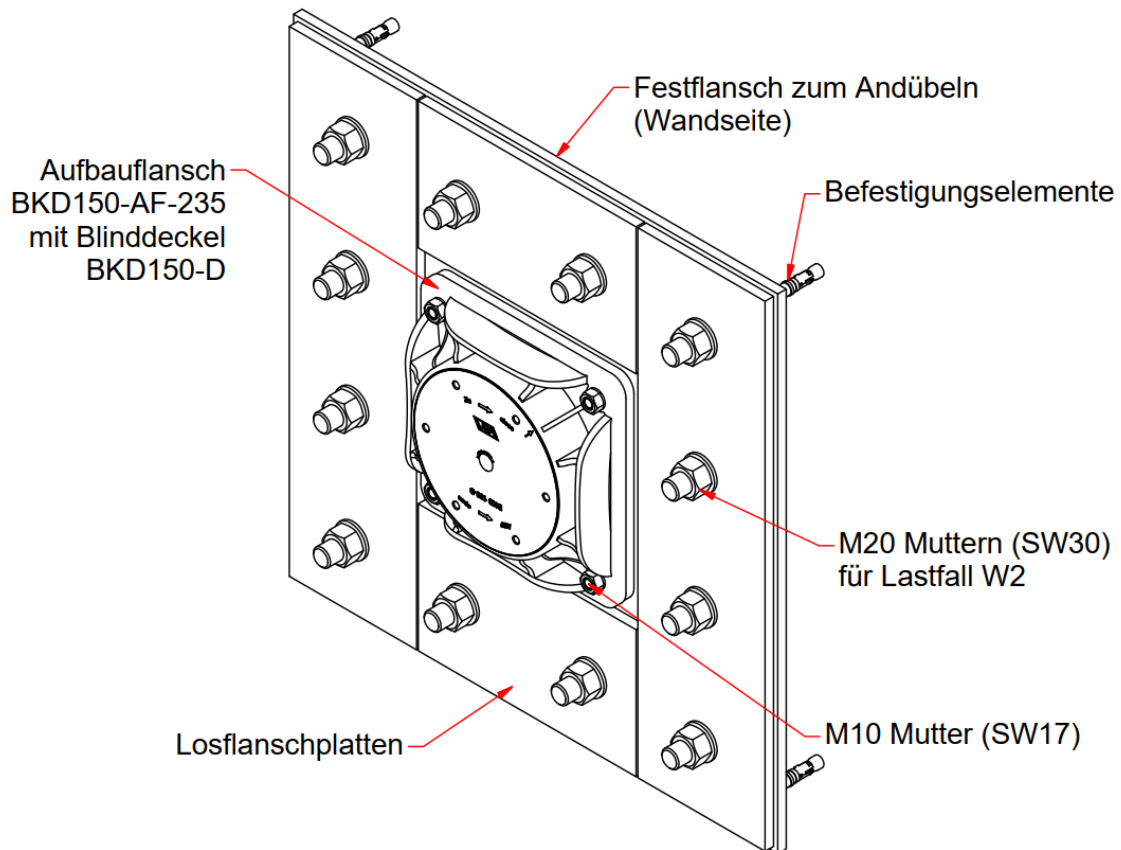
Abbildung 1: Einzelteile der BKD150-AF-NA-F+L-W2/V2A
