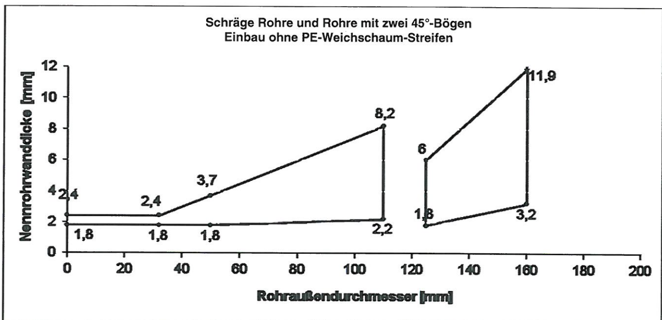
Bild 5 – EI 90-U/C (Deckeneinbau)
