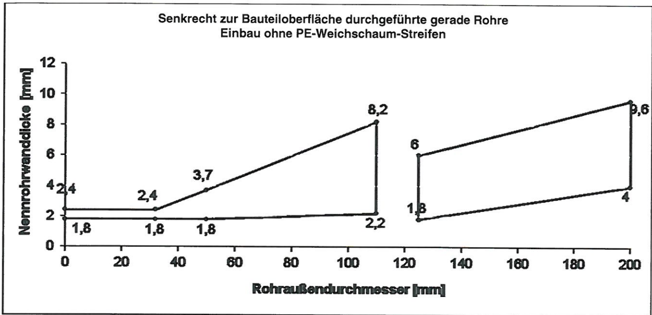
Bild 2 – EI 90-U/C (Wandebau)
