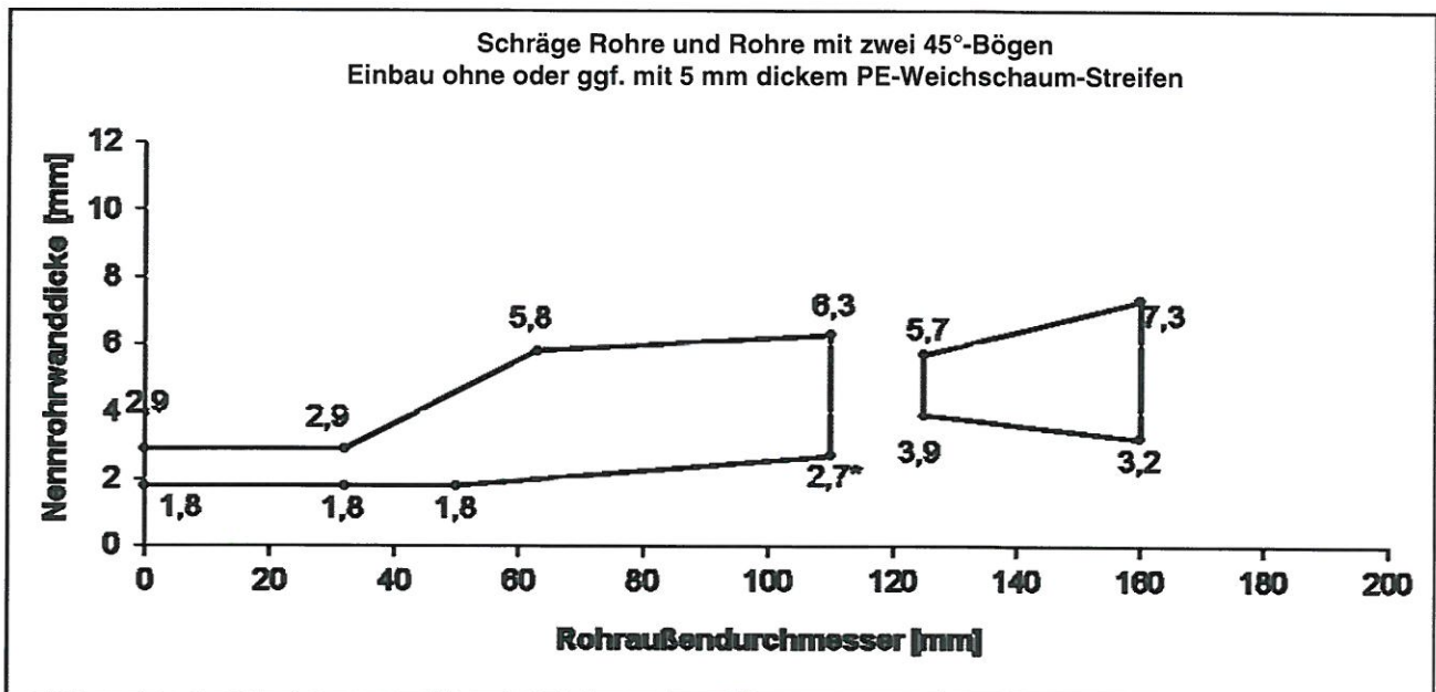
Bild 8 – EI 90-U/C (Wandeinbau)
