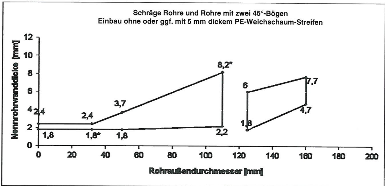
Bild 3 – EI 90-U/C (Wandebau)
