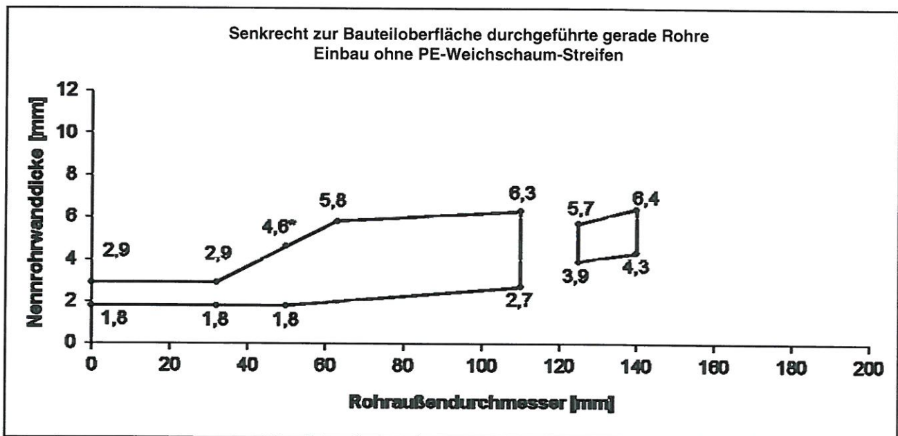
Bild 6 – EI 90-U/U (Wandeinbau)
