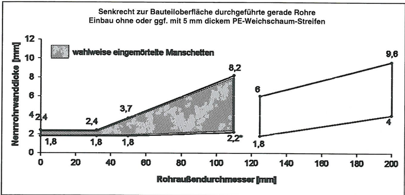
Bild 4 – EI 90-U/C (Deckeneinbau)
