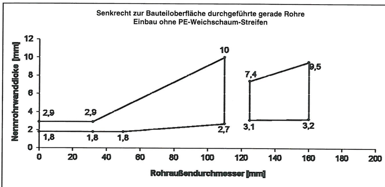
Bild 9 – EI 90-U/U (Deckeneinbau)
