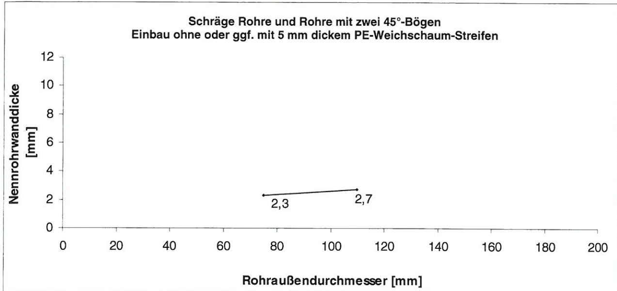
Bild 11 – EI 90-U/U (Deckeneinbau)
