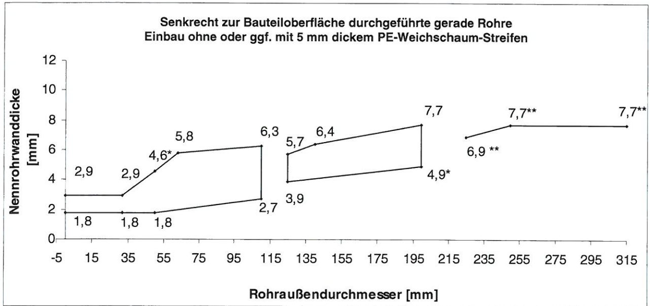
Bild 7 – EI 90-U/C (Wandeinbau)
