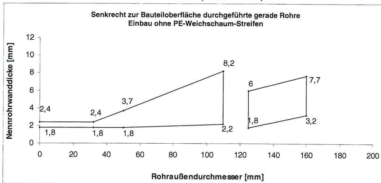
Bild 1 – EI 90-U/U (Wandebau)
