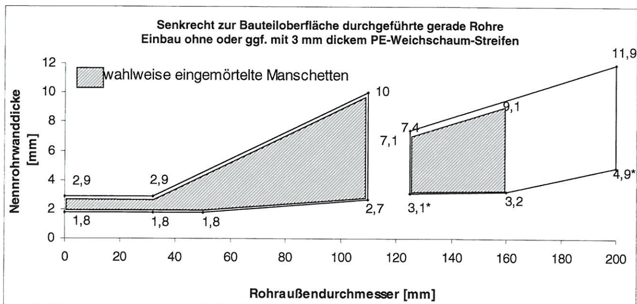
Bild 10 – EI 90-U/C (Deckeneinbau)
