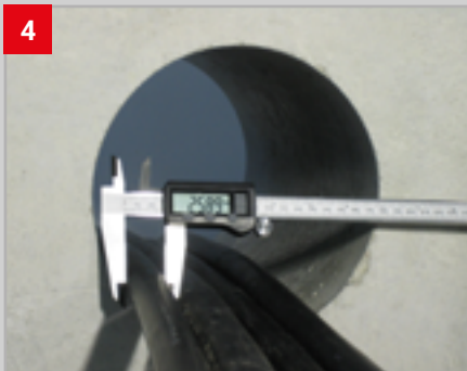
4 Kabeldurchmesser messen!
