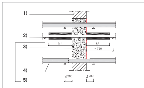
Bild 1: Unterstützung von Rohren und Kabeln / Kabeltragekonstruktionen in Wänden
