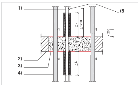
Bild 2: Unterstützung von Rohren und Kabeln / Kabeltragekonstruktionen in Decken
